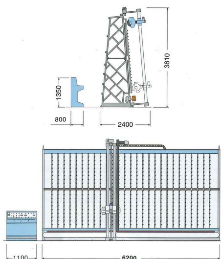
DIMENSIONI (MM)
