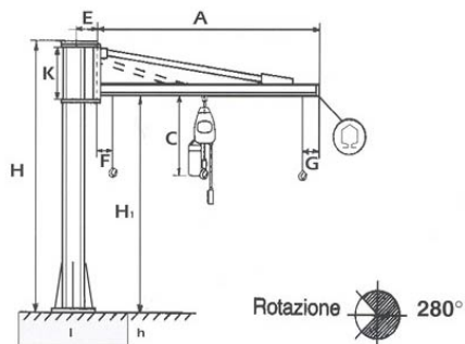
GRU A COLONNA CON BRACCIO IN CANALINA E TIRANTI
