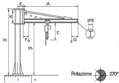
GRU A COLONNA CON BRACCIO IN TRAVE E TIRANTI
