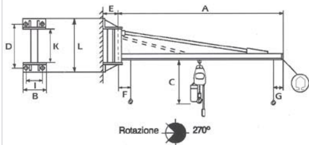
GRU A MENSOLA CON BRACCIO IN CANALINA E TIRANTI
