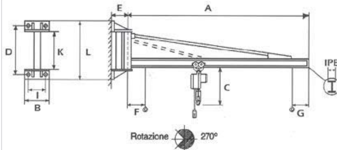
GRU A MENSOLA CON BRACCIO IN TRAVE E TIRANTI
