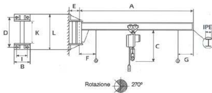
GRU A MENSOLA CON BRACCIO IN TRAVE A SBALZO
